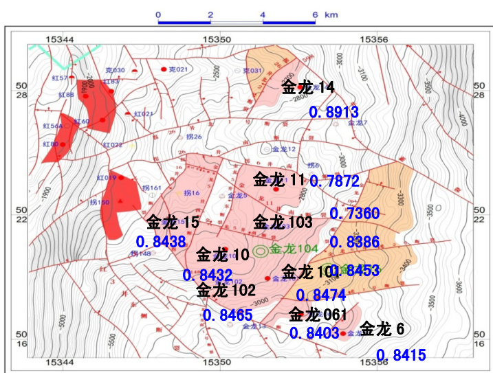
图 1 金龙 10 井区原油密度平面分布图
