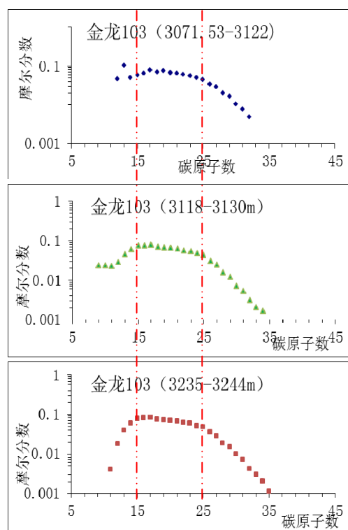
图 2 金龙 103 井正构烷烃含量图
