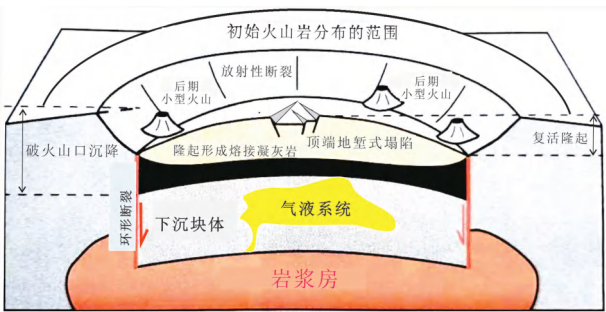
图 2 破火山口形态、构造、岩浆活动特征示意图
