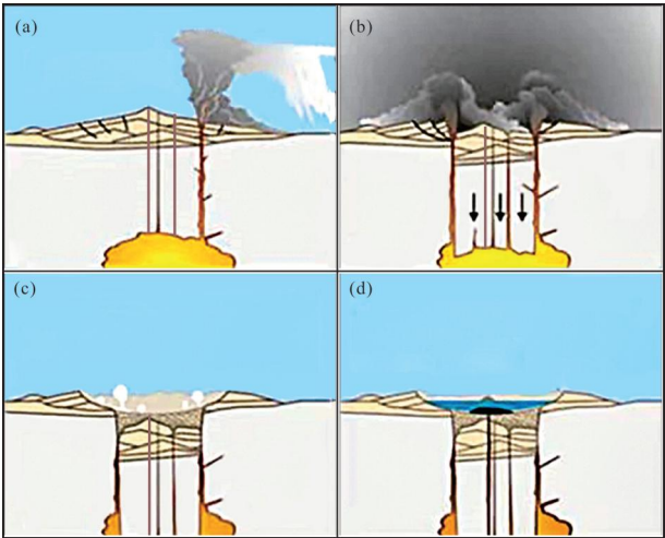
图 3 美国俄亥俄州的 Crater lake 火山口形成示意图(基于 United States Geological Survey, 略有修改): (a) 火山形成后,在侧面又有喷发,酸雨对地区气候有很大影响,此时岩浆房没有大规模持续向上运移岩浆; (b) 岩浆复活阶段,大规模和多点式喷发,掏空岩浆房,造成初始火山崩塌,形成很多的放射和环状断裂; (c) 沿着断裂初始火山形成前后的断裂、塌陷过程形成的放射性和环状断裂,晚期矿化液体充填; (d) 最后有中心或侧翼岩浆侵入,形成小岩株穹窿或矿化穹窿
