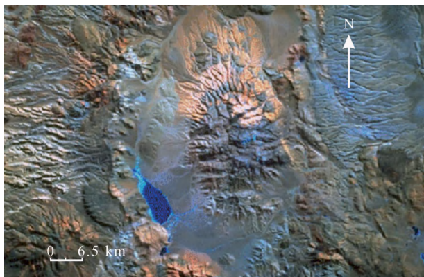
图 5 阿根廷 Cerro Galan 破火山口, 是一个南北方向延展的椭圆形
