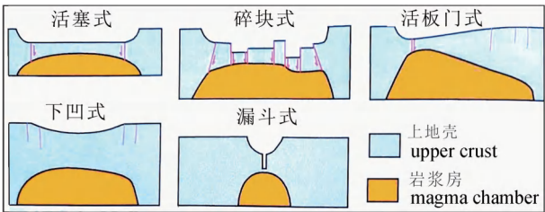
图 1 五种描述破火山口的几何类型 (基于 Acocella, 2021)
